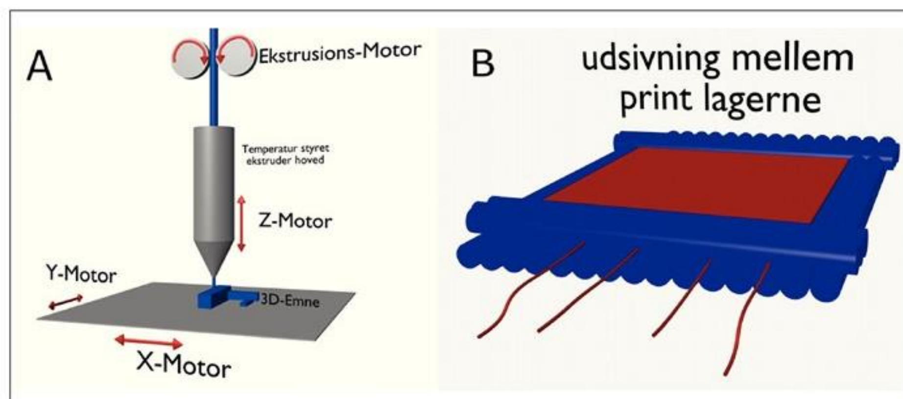
Figur 2. A: Overblik over fused deposition modelling (FDM)-teknologien. Et polymerfilament deponeres vha. ekstruderens motor, der føres igennem det opvarmede ekstruderhovede (225 °C) på en opvarmet arbejdsplatform, der bevæges i x-y-retninger. Selve ekstruderhovedet kan bevæges i z (højde)-retningen. B: Illustrerer et problem i relation til væskehåndtering i printede strukturer. De smeltede filamenter placeres i højere vinkel på hinanden. Mellem hvert enkelt filament opstår en lille spalte, der potentielt giver et hul til udsivning af væske.
