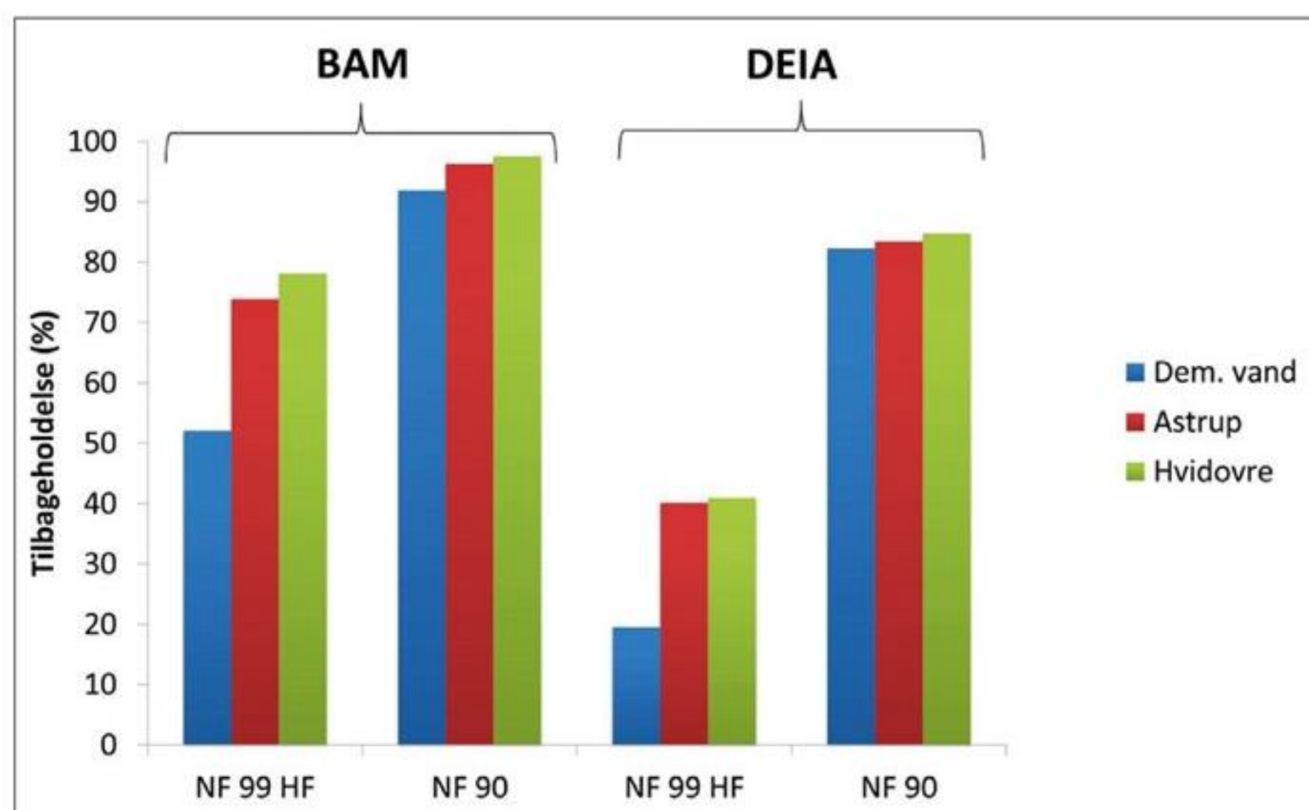
Figur 3. Effekt af grundvand på tilbageholdelse af pesticider.
