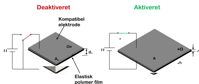
Figur 1. Illustration af princippet bag DEAP aktuator teknologien. Når en spænding tilføres til elektroderne, vil de elektrostatisk kræfter presse elastomeren sammen og filmen vil udvide sig i planet på grund af materialets inkompressibilitet. Når den eksterne spænding slås fra, vender materialet tilbage til sin oprindelige form.
