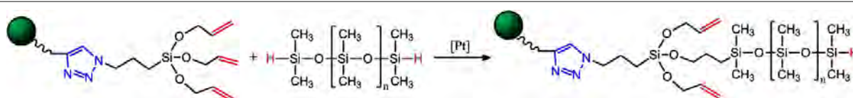
Figur 10. Hydrosilyleringsreaktion mellem vinylgrupperne på krydsbinderen og hydrid-endergrupper på polydimethylsiloxane (PDMS), en siliconepolymer.
